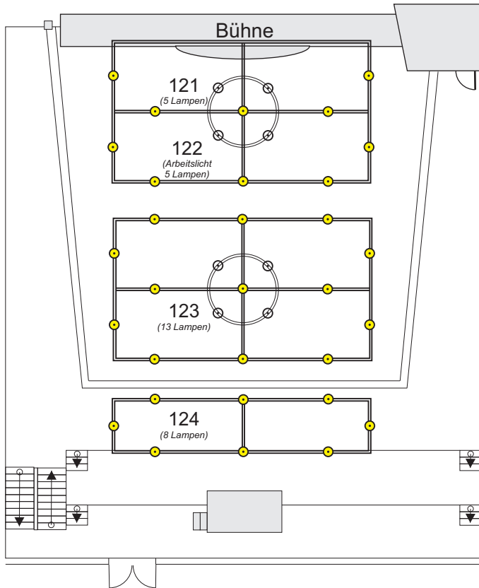
● Lampen hängende Montage
