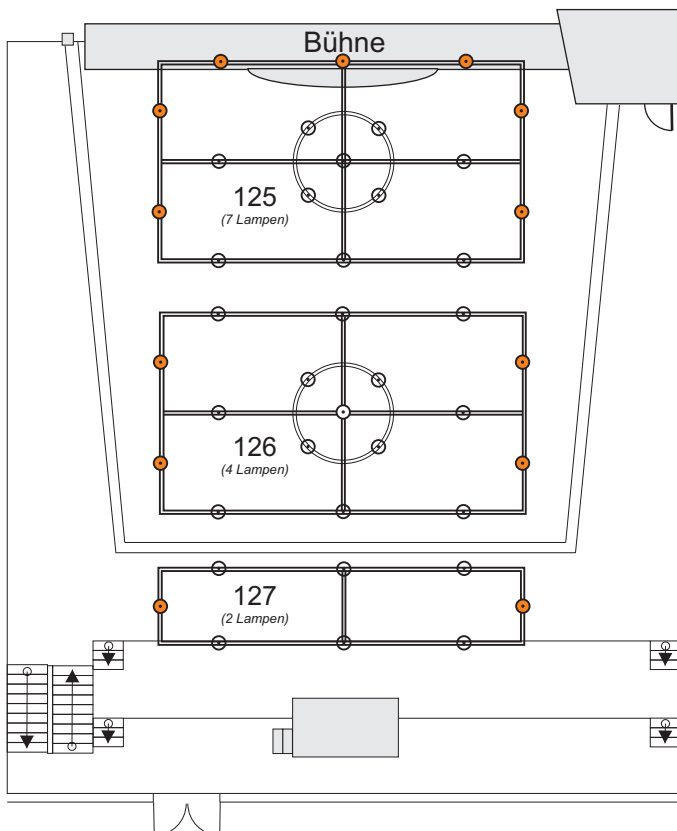
● Lampen stehende Montage
